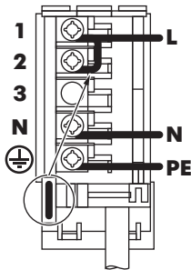
Conexión monofásica 220 V - 240 V ~
