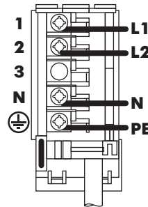
Conexión bifásica 400 V 2L-1N ~
